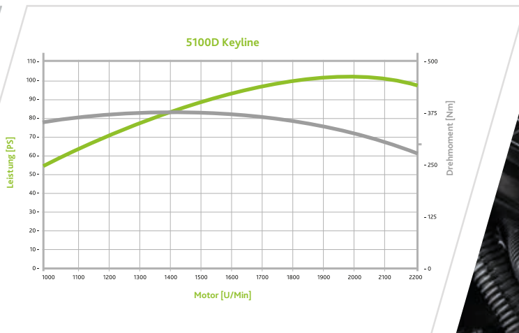
> Leistungsdiagramm 5100D Keyline.
